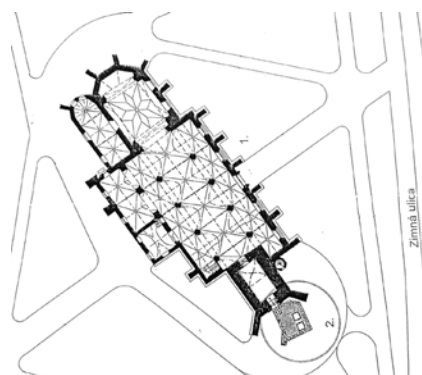
Pôdorys farského kostola (zdroj – F. Javorský, štúdia)
